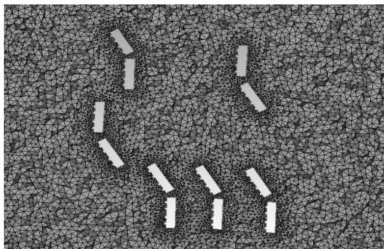
شکل ۶. شبکه‌بندی ساختاریافته در دامنه محاسباتی بر مبنای بررسی استقلال حل از شبکه به تعداد ۷۰۱۰۰۹۴
