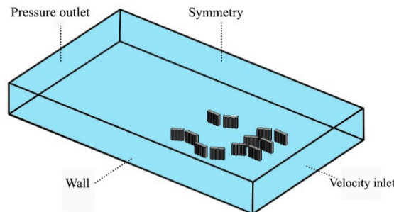
شکل ۳. شرایط مرزی دامنه محاسباتی
