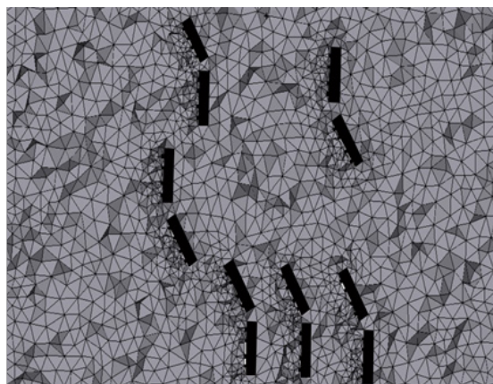
(الف) مش درشت (تعداد مش: ۵,۶۲۰,۷۰۱)
