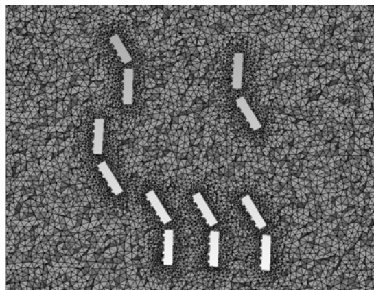
(ج) مش ریز (تعداد مش: ۱۰,۱۵۸,۷۴۶)
